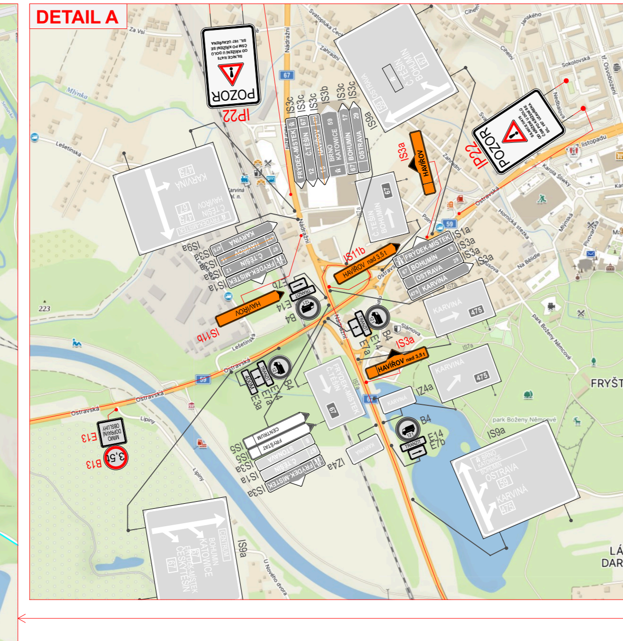
DETAIL MÍSTA ÚPRAVY
